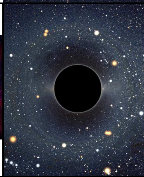
trou noir
