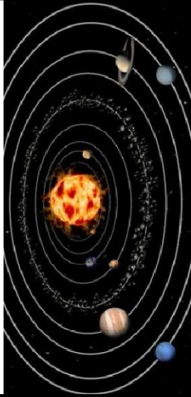
systeme solaire
